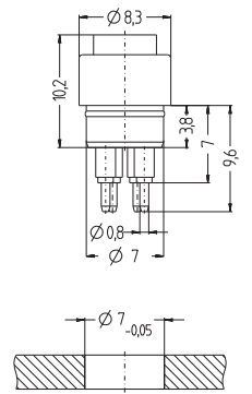
EKP_print-contact
