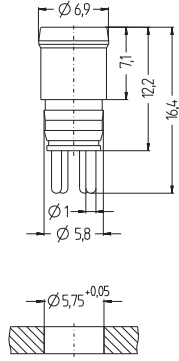
ESP_print-contact
